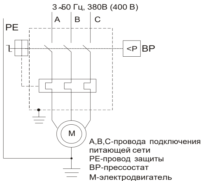
Рисунок А.1 - Схема электрическая принципиальная компрессоров СБ4/С-100.AB858, СБ4/С-270.AB858, СБ4/Ф-270.AB858, СБ4/Ф-270.AB858В, СБ4/Ф-500.AB858, СБ4/Ф-270.AB858/16, СБ4/Ф-500.AB858/16
