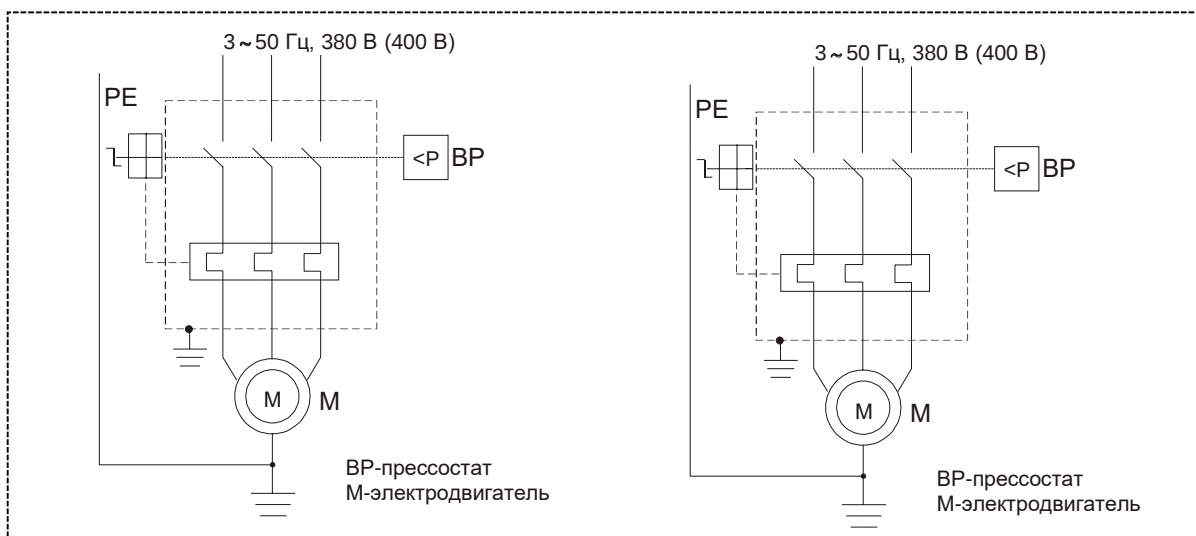
Рисунок А.2 – Схема электрическая принципиальная компрессора СБ4/Ф-500.AB858ТБ
