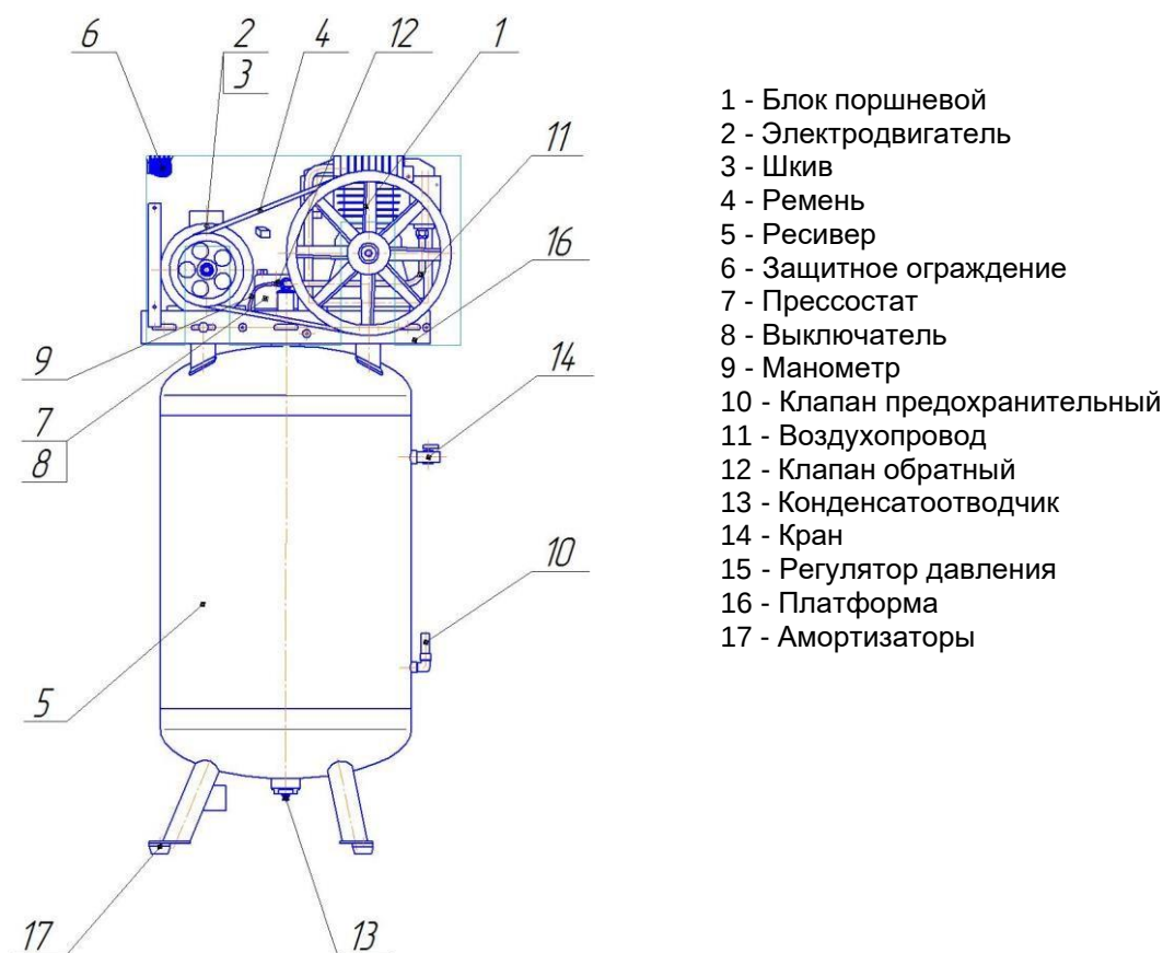
Рисунок 7 - Общий вид компрессора СБ4/Ф-270.АВ858Б
