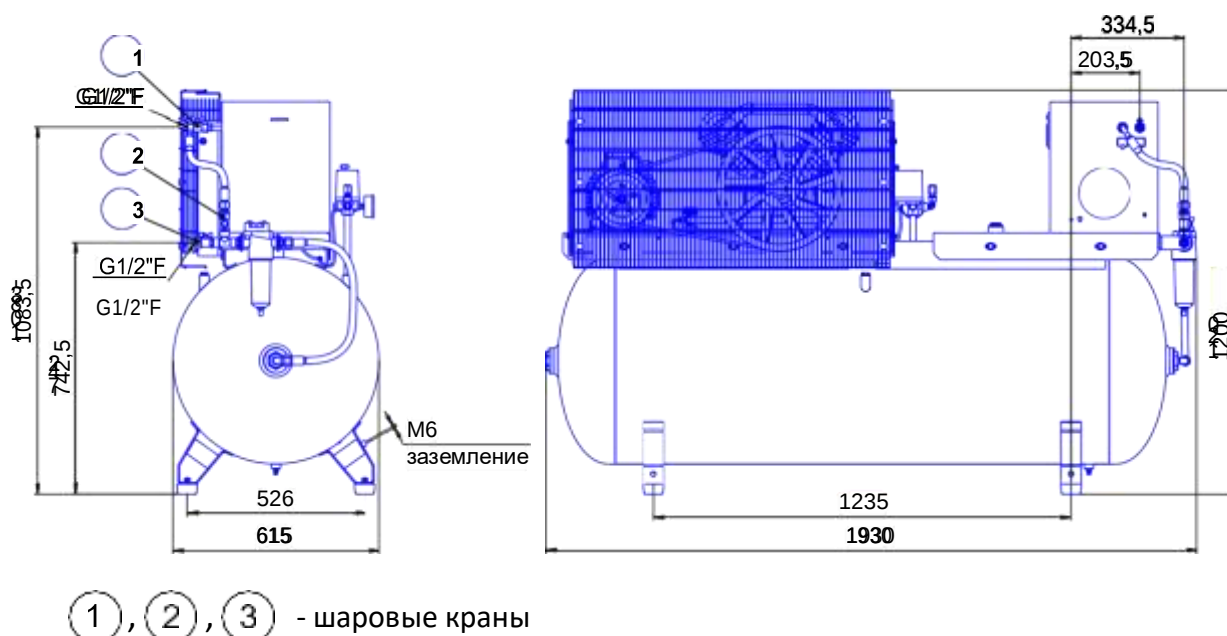
Рисунок 6 - Габаритные и присоединительные размеры компрессора СБ4/Ф-500.LB50Д
