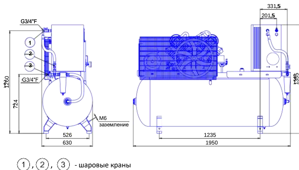
Рисунок 8 - Габаритные и присоединительные размеры компрессора СБ4/Ф-500.LT100Д
