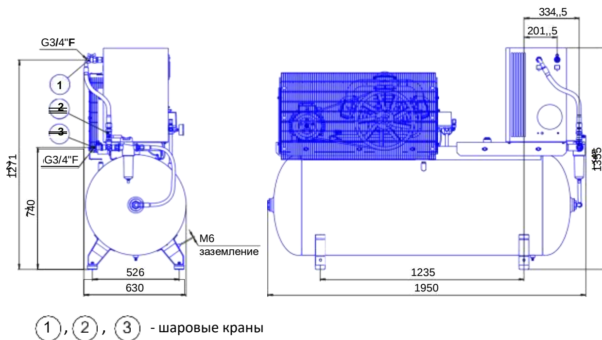
Рисунок 7 - Габаритные и присоединительные размеры компрессора СБ4/Ф-500.LB75Д
