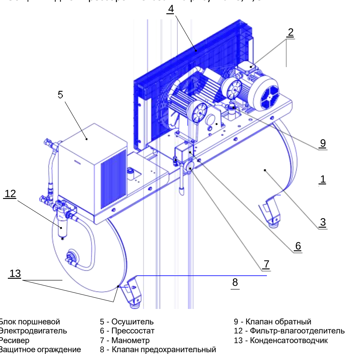
Рисунок 3 - Общий вид компрессора CB4/Φ-500.LB50D
