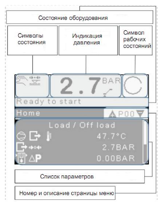
Рис. 1. Дисплей контроллера
