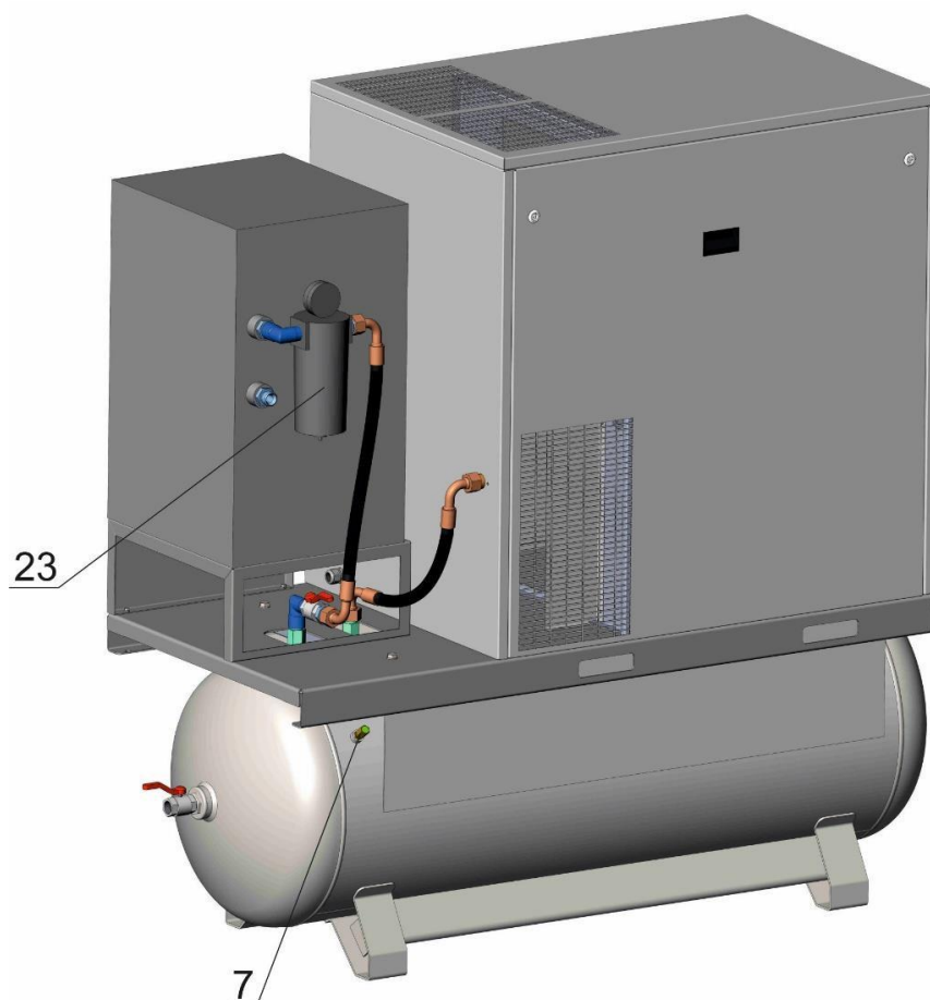
Рисунок 3 – Общий вид компрессорных установок ВК25-...-500Д(BC), ВК30-...-500Д(BC)
