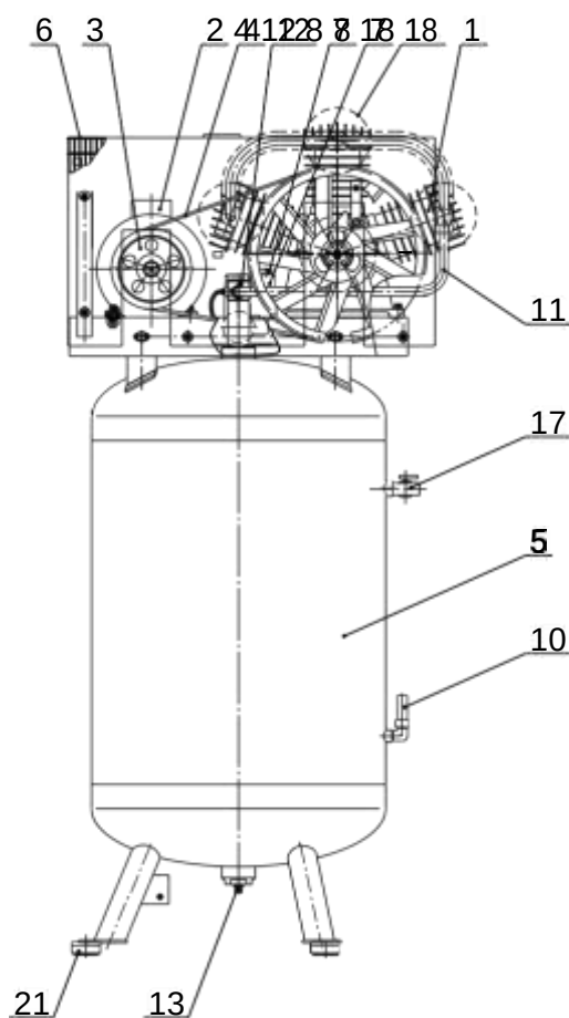
Рисунок 6 - Общий вид компрессора СБ4/Φ-270.LB75B
