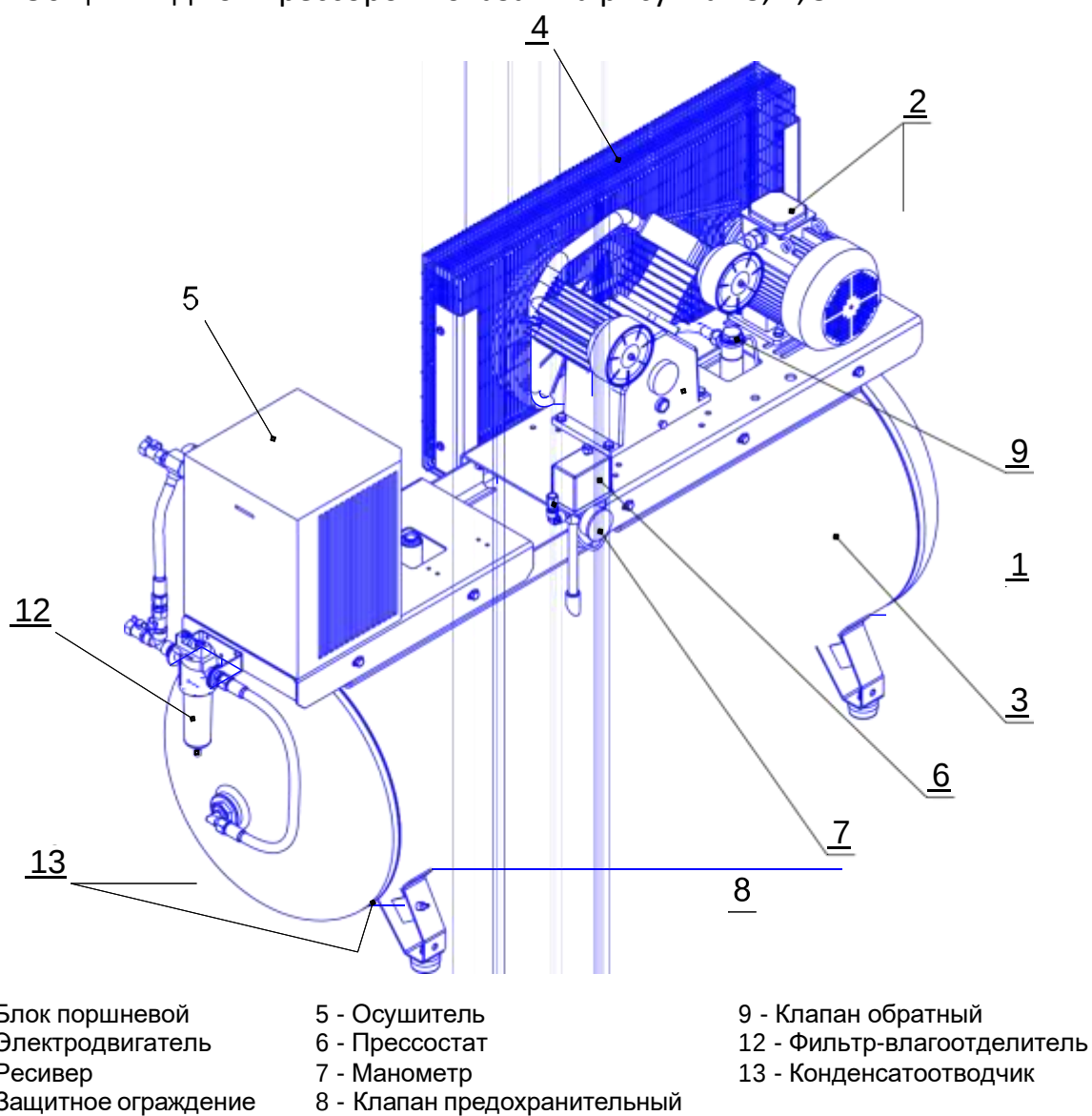
Рисунок 3 - Общий вид компрессора СБ4/Ф-500.LB50Д
