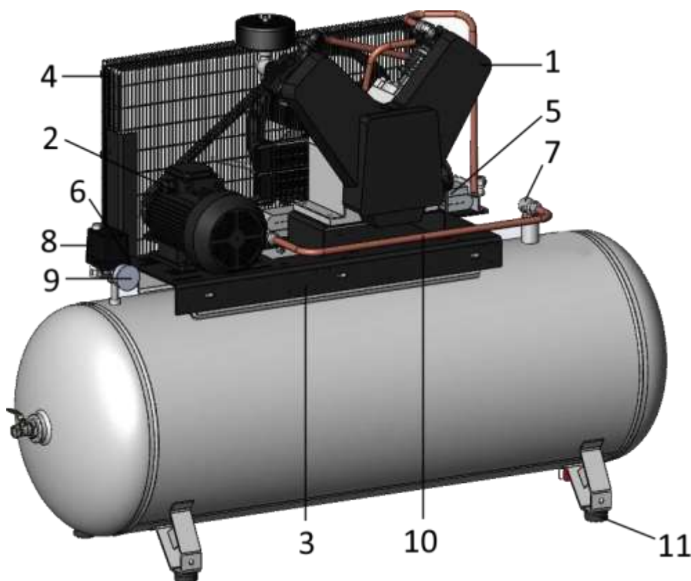
Рисунок 3 Установка компрессорная СБ4-500.F55/8, СБ4-500.F55, СБ4-500.F55/14
