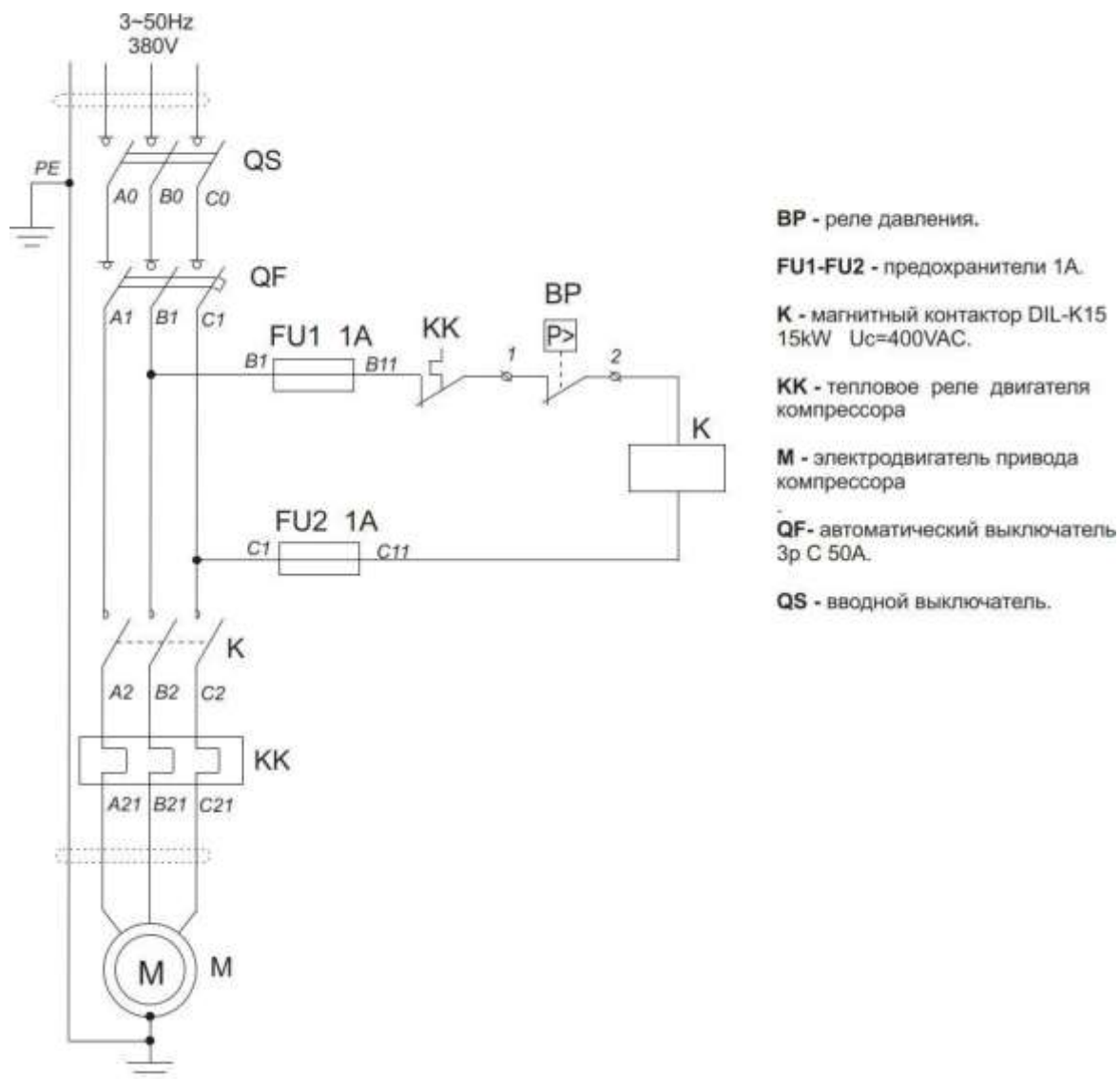
Рисунок А.1 - Схема электрическая принципиальная компрессоров СБ4-500.F55, СБ4-500.F55/14
