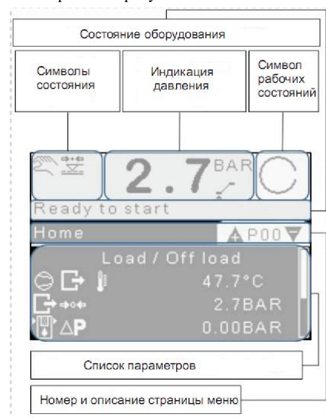
Рис. 1. Дисплей контроллера
