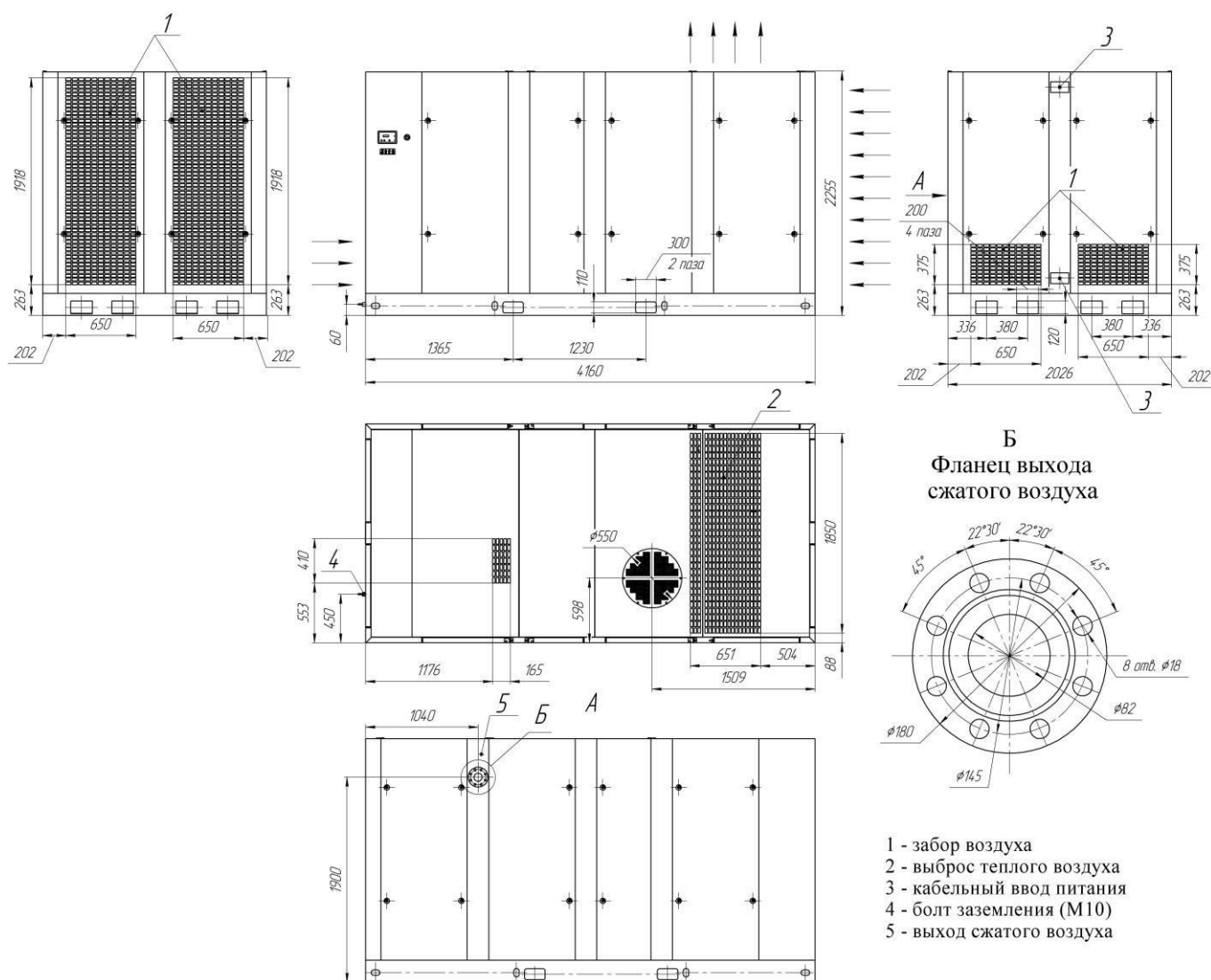
Рисунок А.1 Габаритные и присоединительные размеры компрессорной установки BK430-7,5H (BK430-7,5BC)
