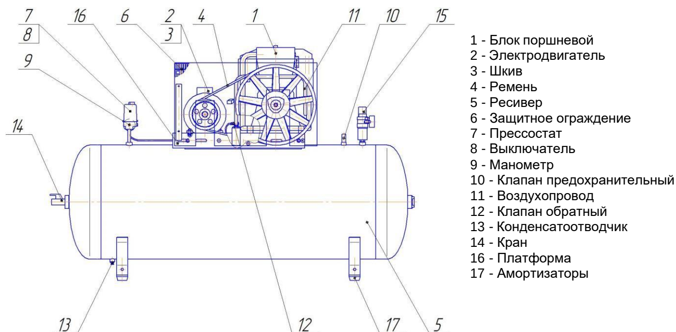
Рисунок 3 - Общий вид компрессора СБ4/Ф-500.AB998
