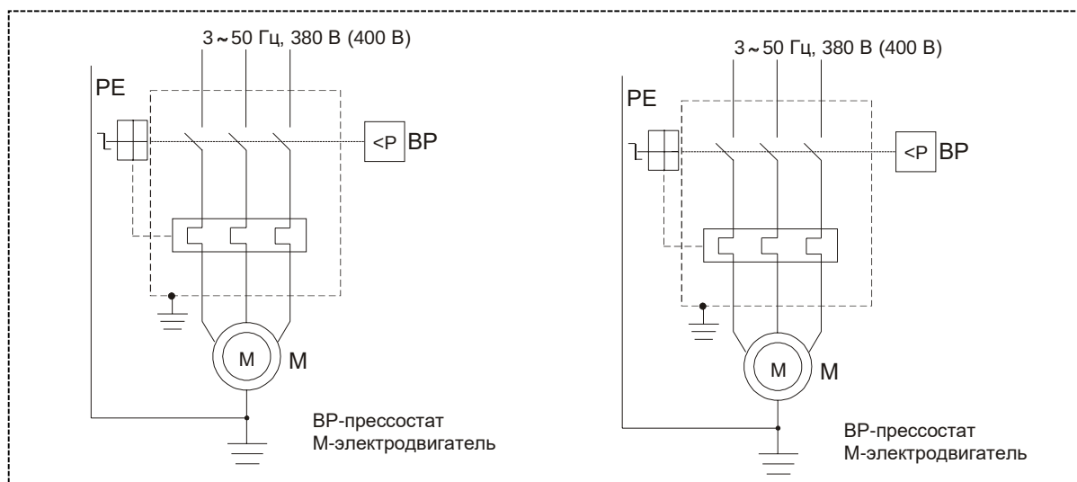
Рисунок А.2 – Схема электрическая принципиальная компрессора СБ4/Ф-500.АВ858Т5
