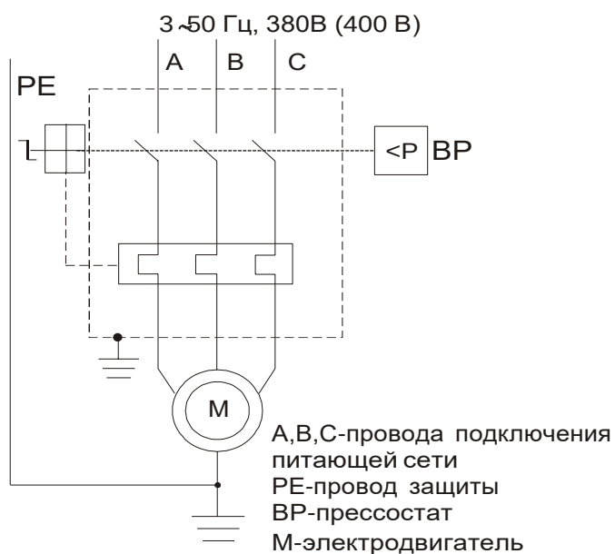
Рисунок А.1 - Схема электрическая принципиальная компрессоров CB4/C-100.AB678, CB4/C-270.AB678, CB4/Ф-270.AB678, CB4/Ф-270.AB678B, CB4/Ф-500.AB678
