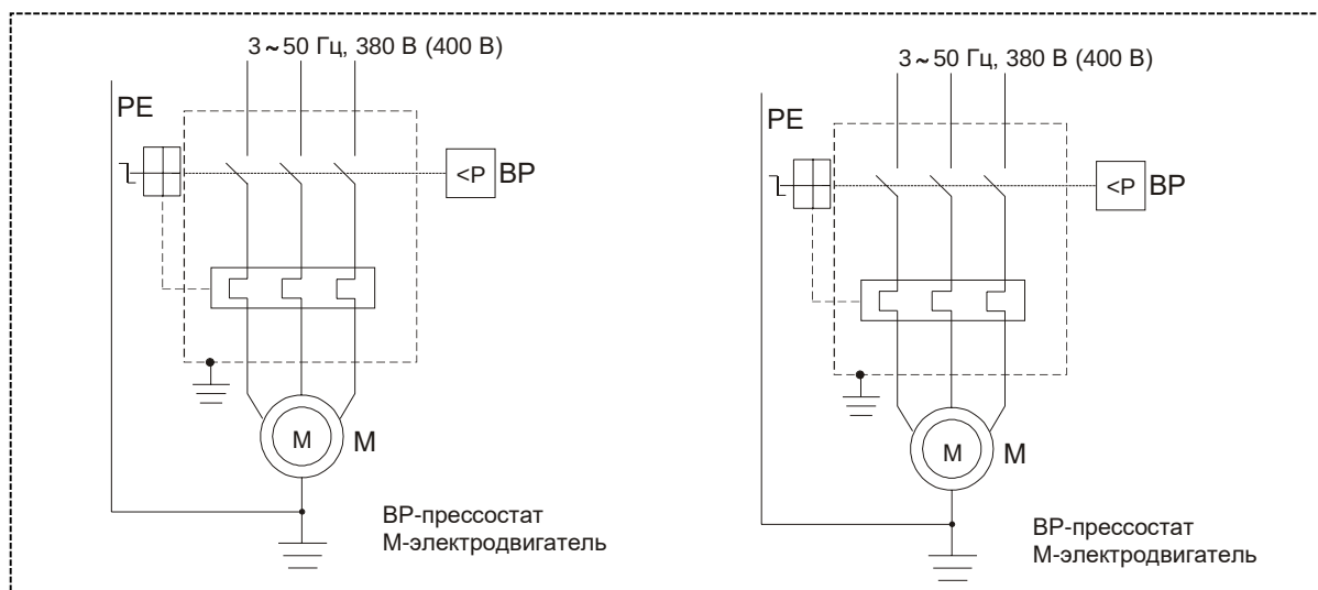
Рисунок А.2 – Схема электрическая принципиальная компрессора CB4/Ф-500.AB678TБ
